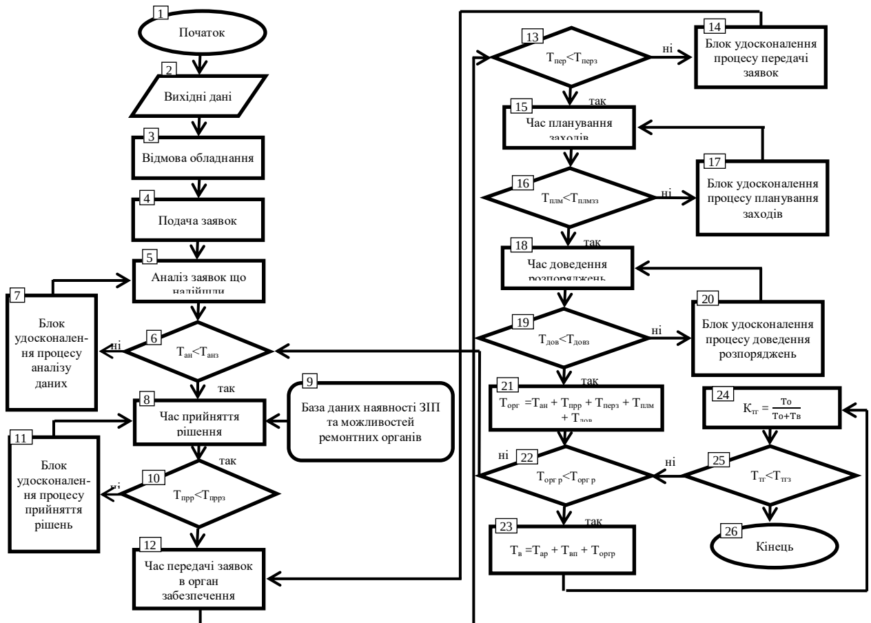
Рисунок 2. Блок-схема методики оцінювання ефективності управління відновленням РЕТ РТВ
