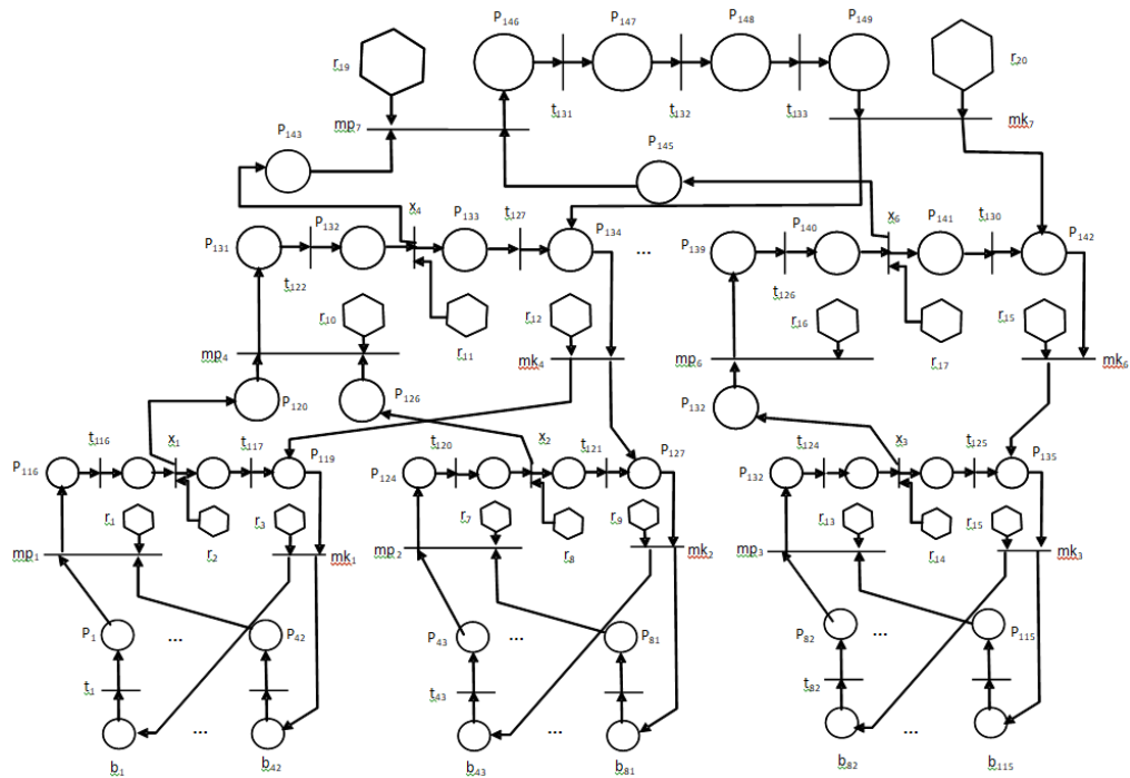
Рисунок 1. Е-мережа управління відновленням РЕТ РТВ
